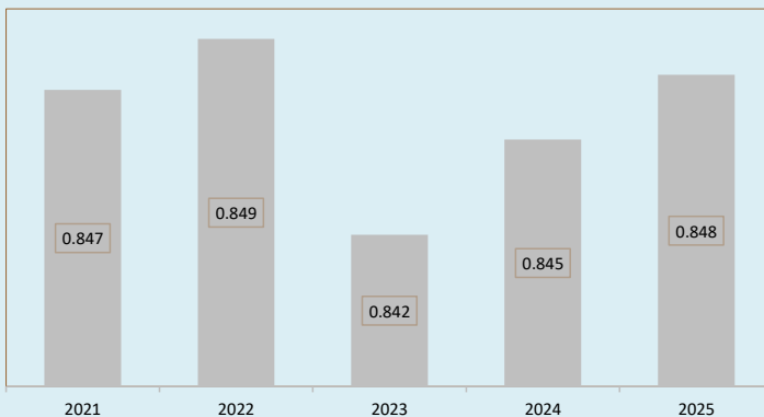
Norma e Varësisë së Sistemit në vite
