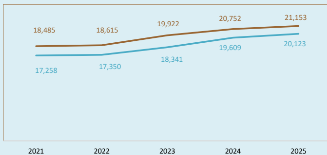
Pensioni mesatar dhe të ardhurat mesatare në vite
